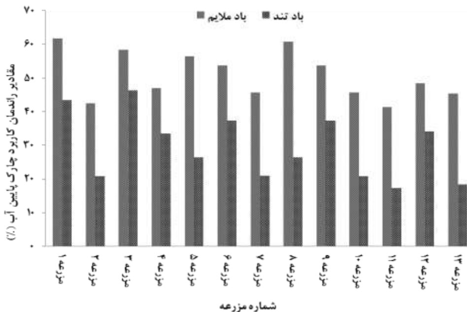
شکل (۳): مقادیر راندمان کاربرد چارک پایین آب در سامانه‌های مورد مطالعه
