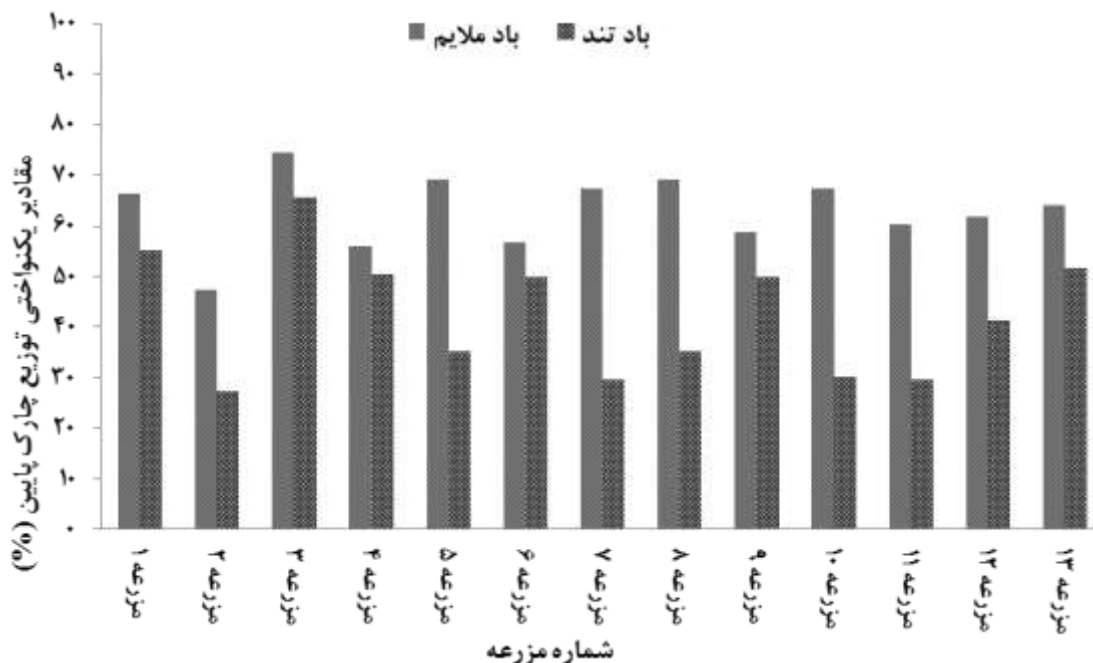
شکل (۲): مقادیر یکنواختی توزیع چارک پایین آب در سامانه‌های مورد مطالعه
