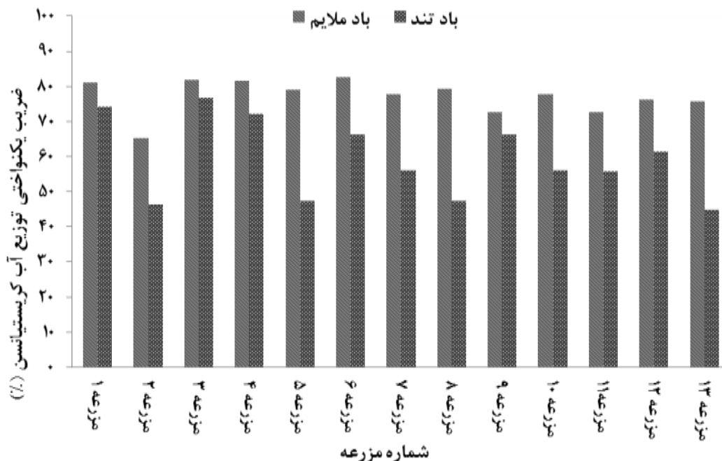
شکل (۱): مقادیر ضریب یکنواختی توزیع آب کریستیانسن سامانه در مزارع مورد مطالعه
